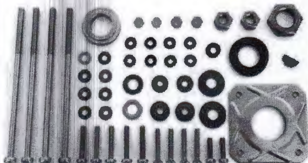
REPARO DO ALTERNADOR REPARO DO ALTERNADOR BOSCH KCB1 80A, MERCEDES "ELETRÔNICO"
