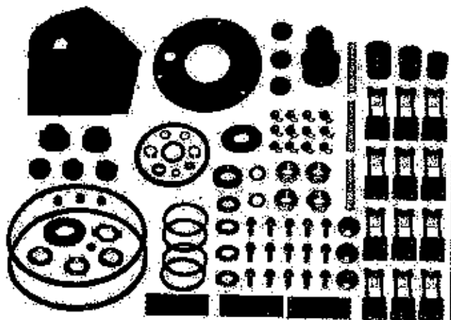
REPARO PARTIDA PARTIDA DELCO REMY 50MT 24V 12 ESCOVAS COMPLETO CATERPILLAR - CLARK - CUMMINS
