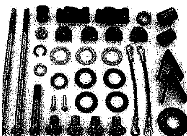
REPARO PARTIDA DELCO C10 C10X OPILA COMPLETO C10X FIX C10 PORTA ESCOVAS
