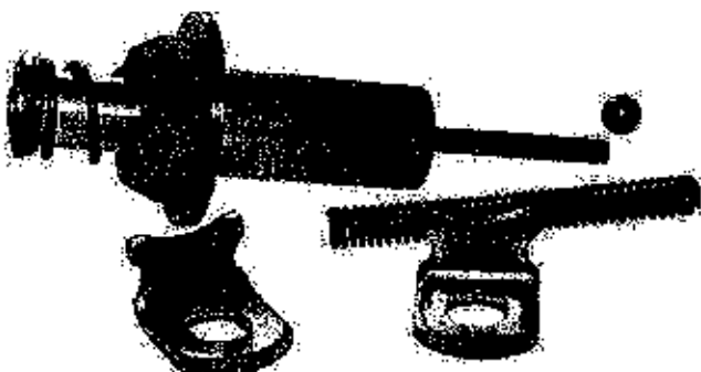
REPARO PARTIDA REP. PISTÃO CILINDRO FICHAVE MAG. AUTOMÁTICO TOPICORSTA (PARTIDA NIPPONDEN- SO 10MM)
